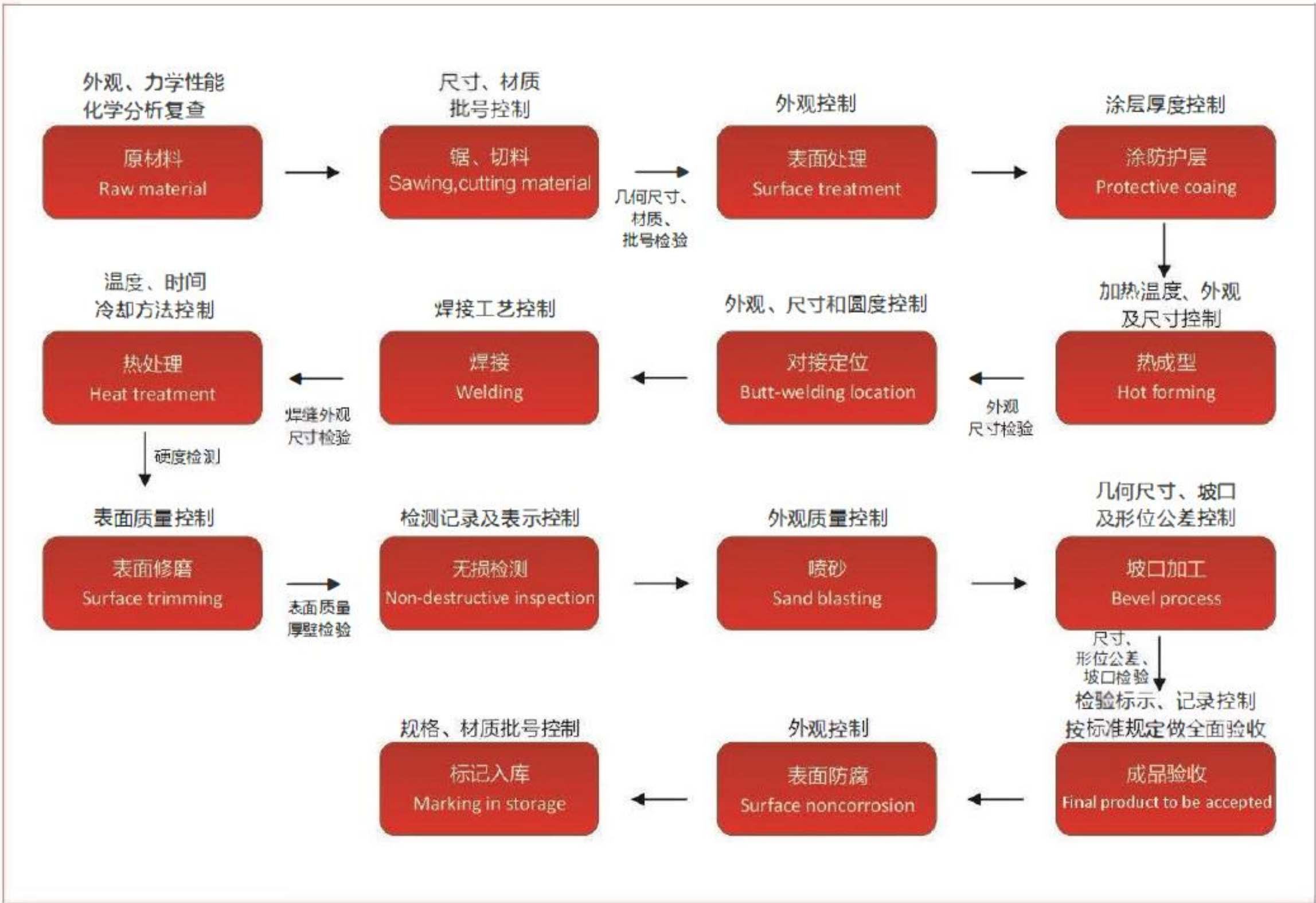
无缝碳钢、合金管件工艺流程图（热成型）
