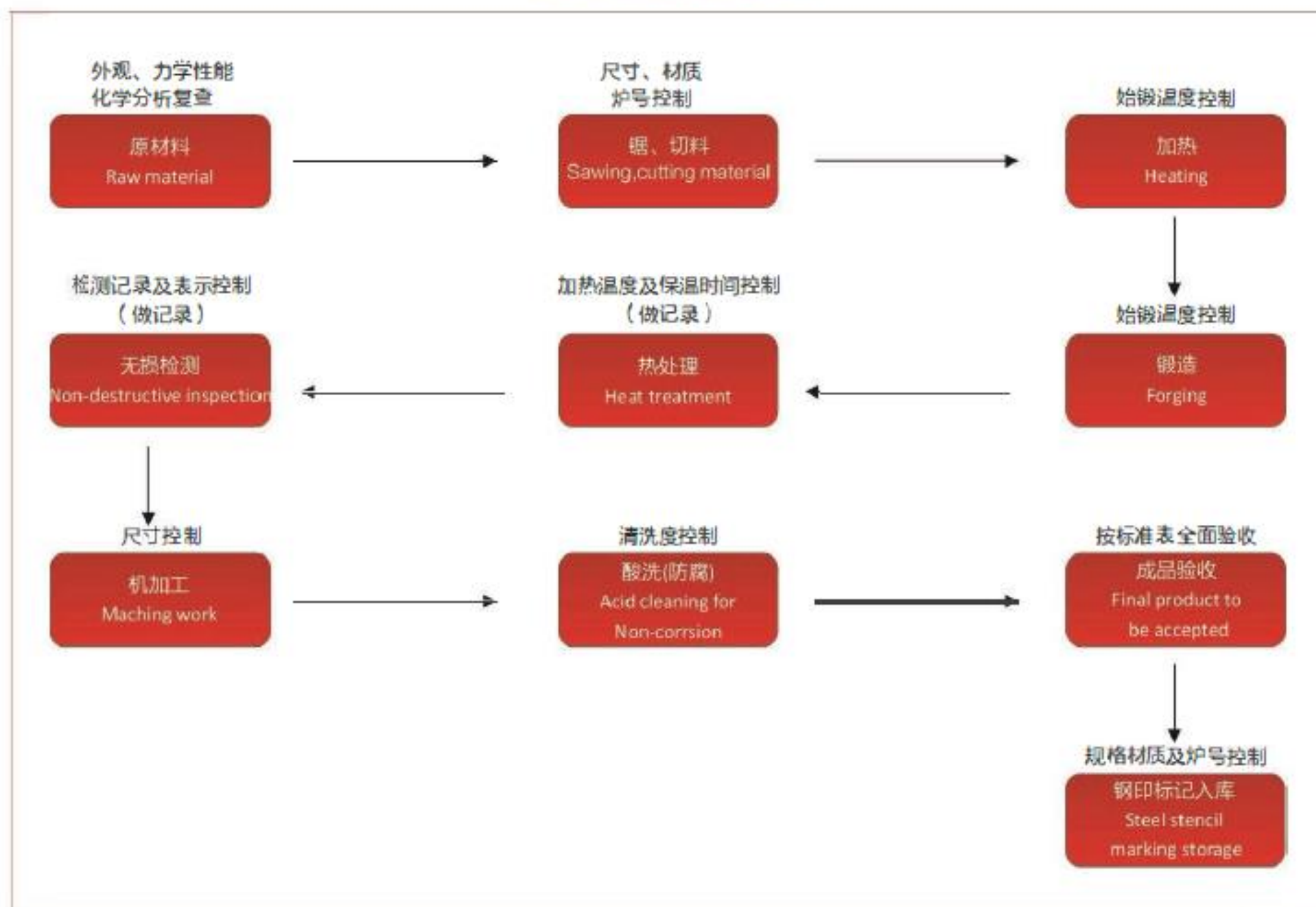
锻造法兰工艺流程图
