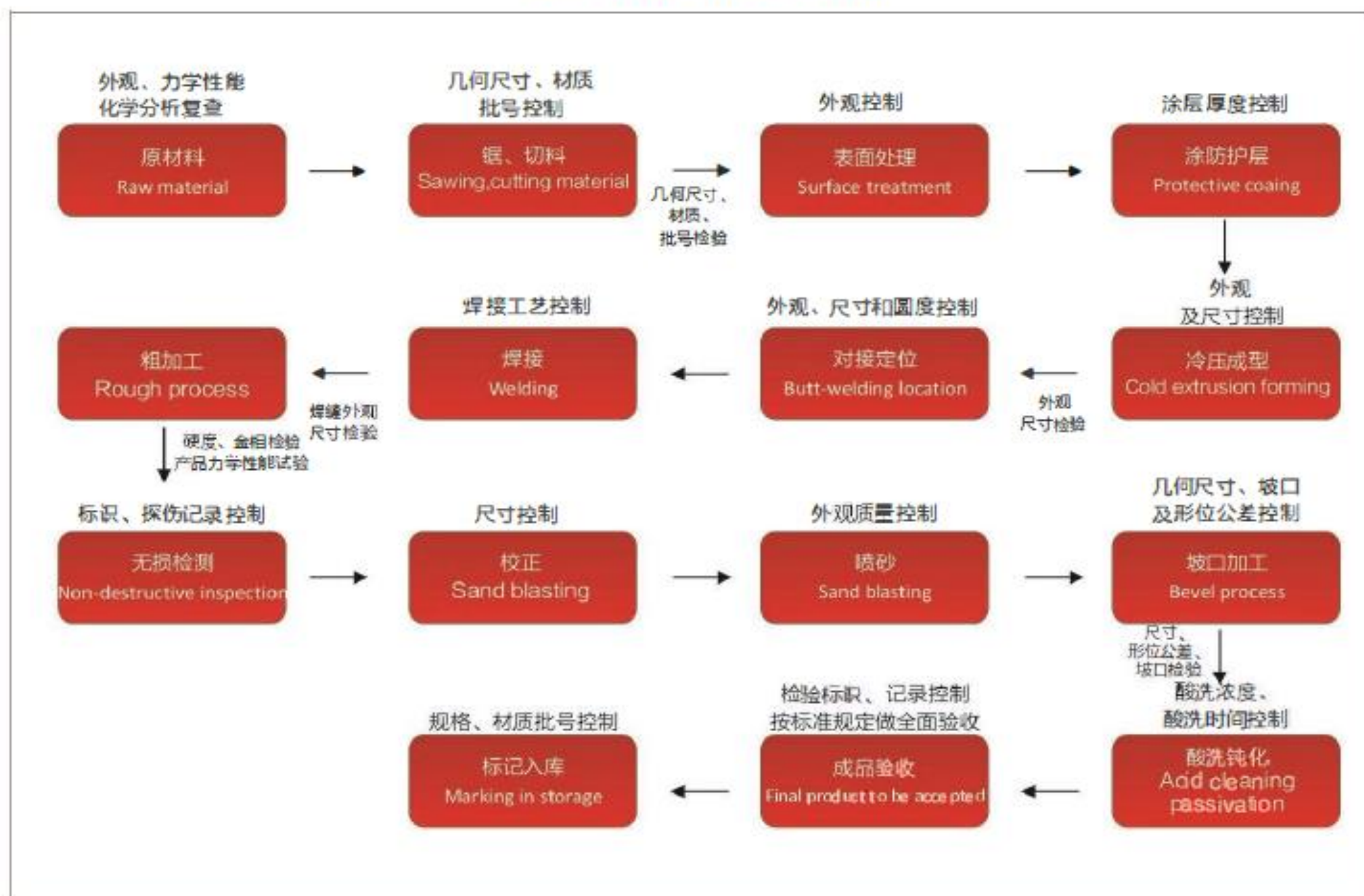
板制不锈钢管件工艺流程图
